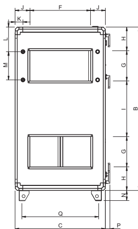
Topvex SC06
