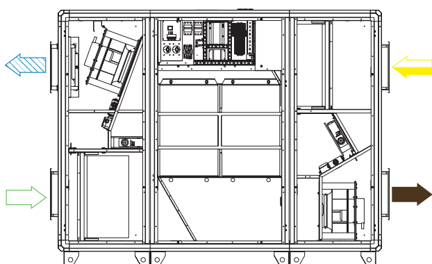
Левосторонний агрегат
