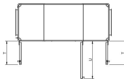
Вид сверху. Левосторонний агрегат
