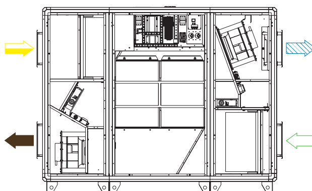
Правосторонний агрегат
